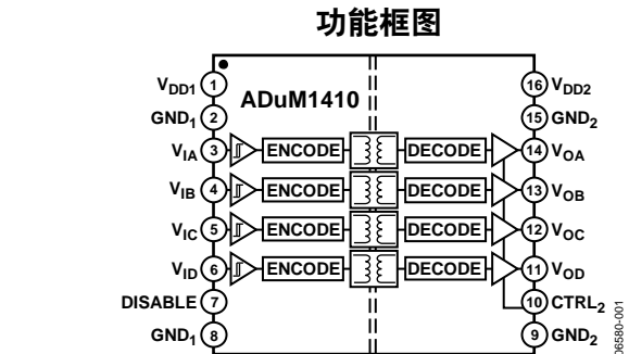
图1. ADuM1410
