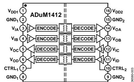
图3. ADuM1412
