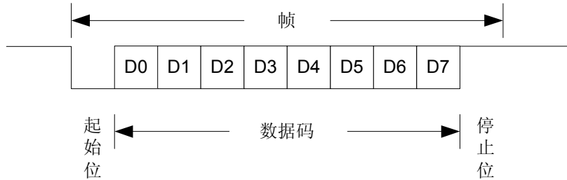
图 5-22 UART1 8 位数据格式
