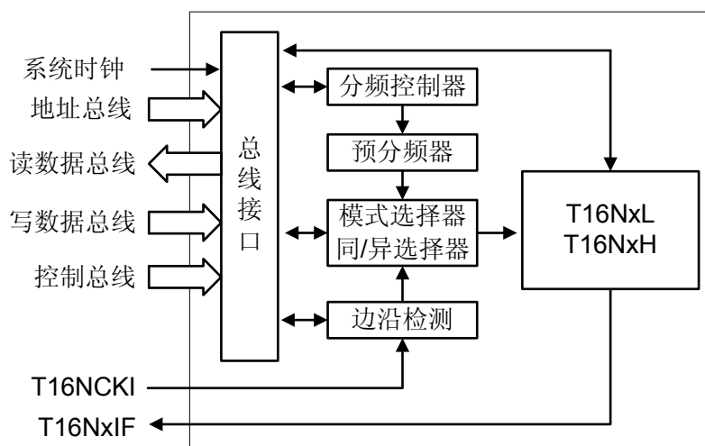
图 5-3 T16Nx 内部结构图
