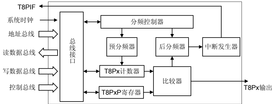
图 5-2 T8Px 内部结构图
