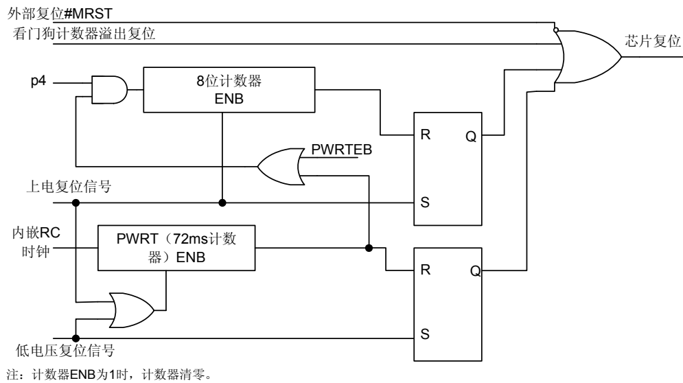
图 6-2 芯片复位原理图
