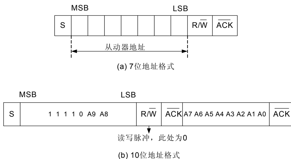
图 5-18 地址发送示意图
