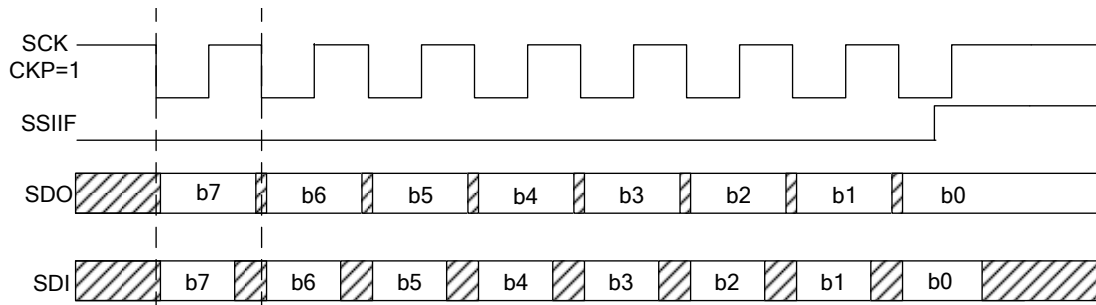
图 5-12 SPI 主控模式时序图 (CKP = 1)
