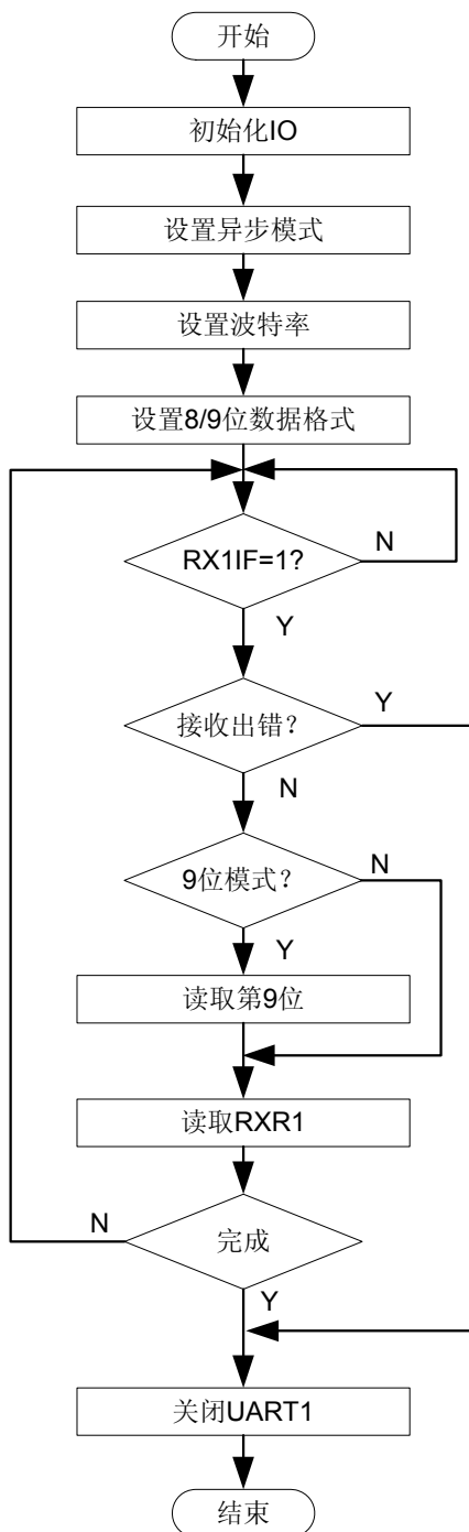
图 5-25 UART1 接收器流程图
