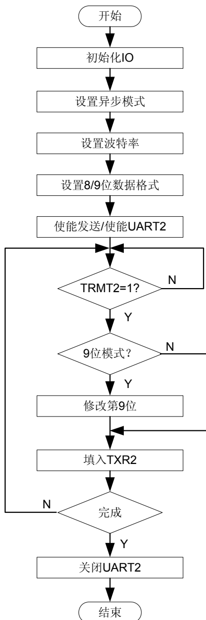
图 5-31 UART2 发送器流程图
