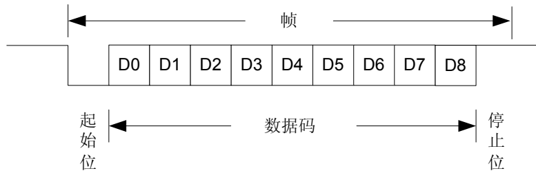
图 5-23 UART1 9 位数据格式
