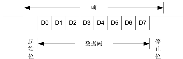
图 5-29 UART2 8 位数据格式
