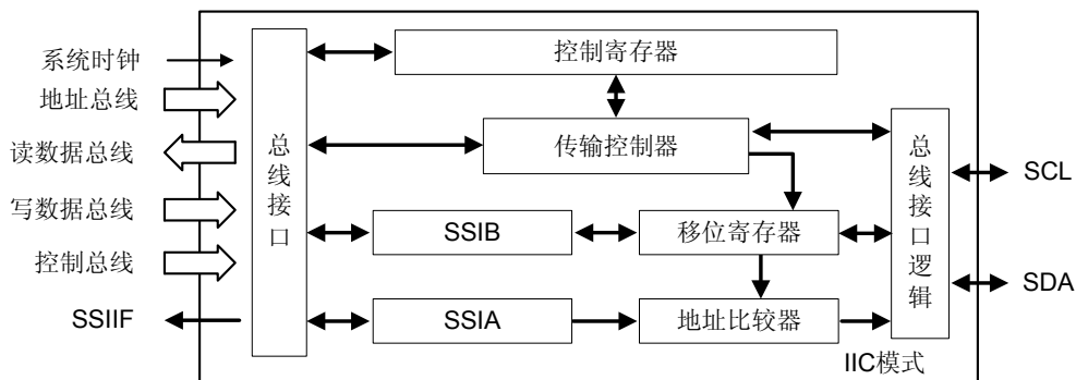
图 5-17 IIC 模式结构框图
