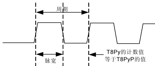
图 5-7 PWM 输出示意图
