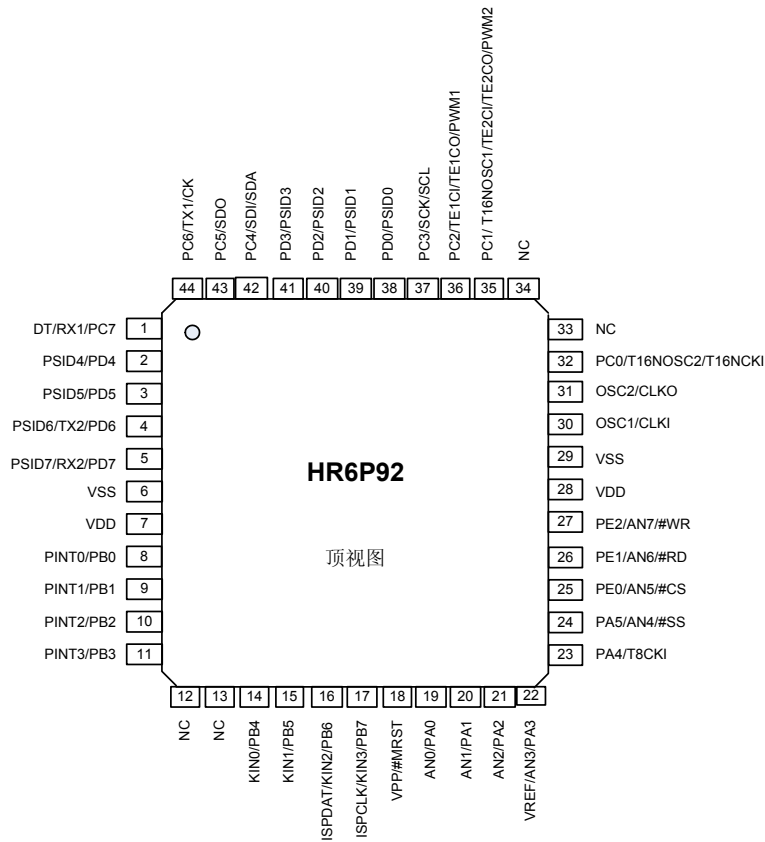
图 1-5 HR6P92/92H (LQFP44) 顶视图
