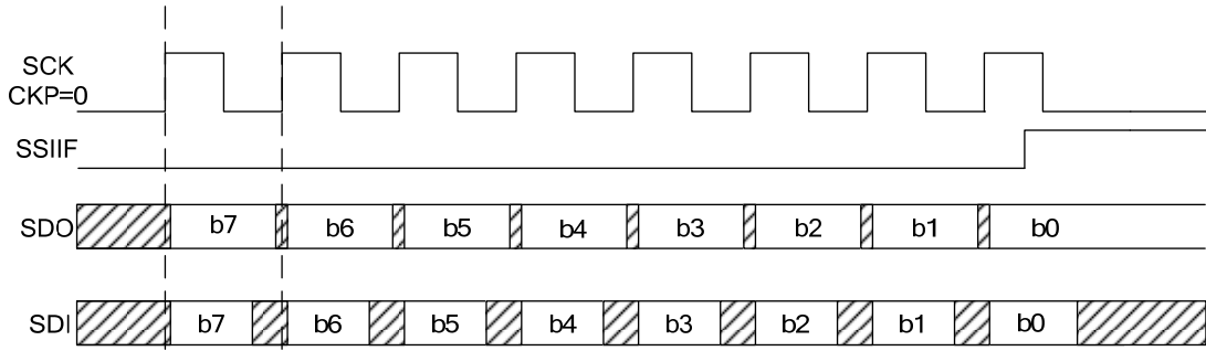
图 5-13 SPI 主控模式时序图 (CKP = 0)
