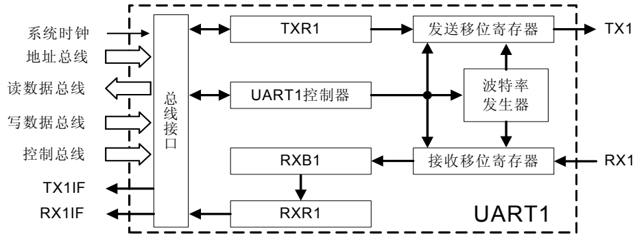
图 5-21 UART1 结构框图
