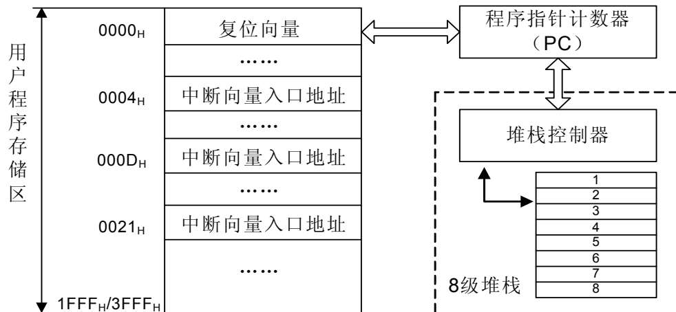
图 3-1 程序区地址映射和堆栈示意图
