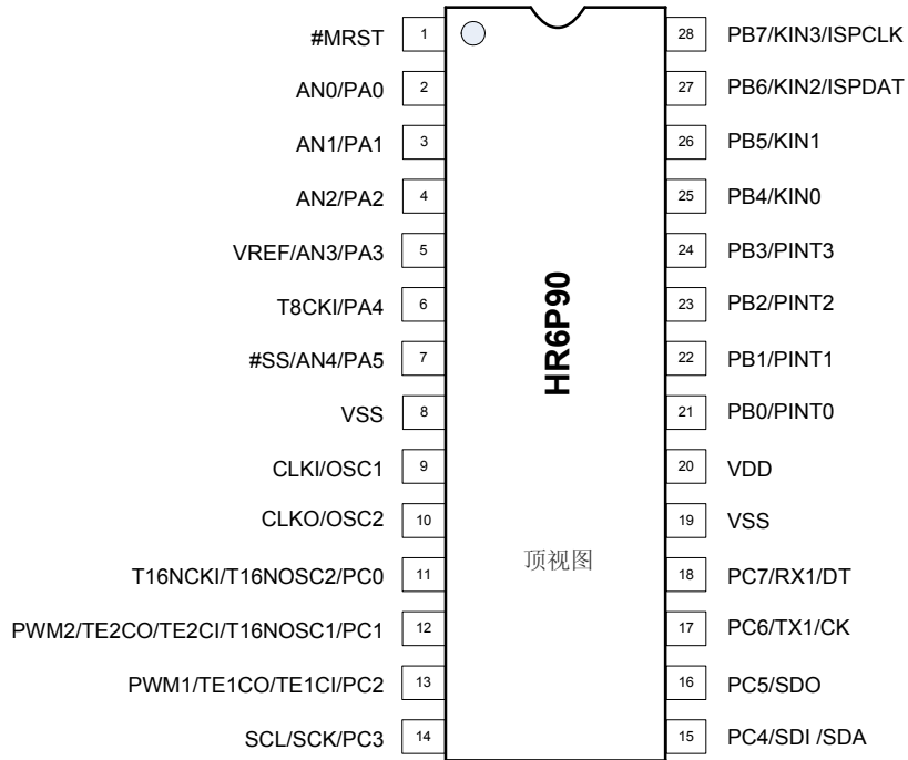
图 1-2 HR6P90/90H (SKDIP28/SOP28) 顶视图
