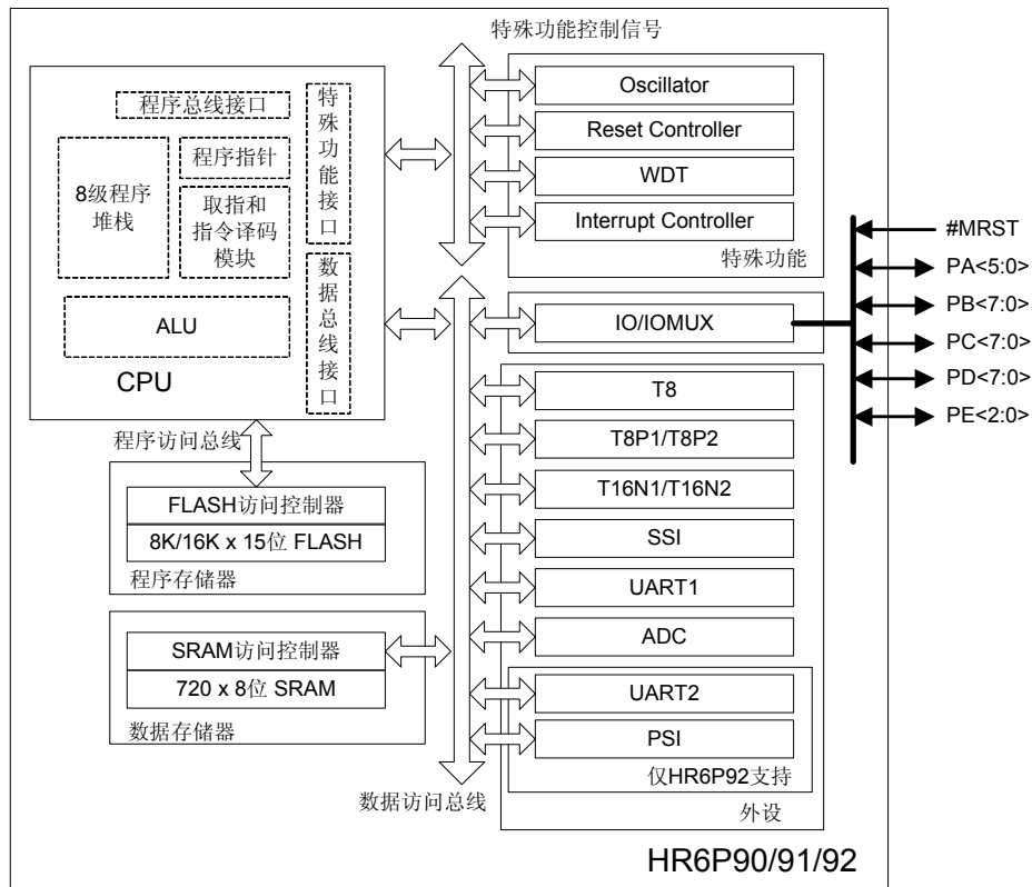
图 1-1 HR6P90/90H/91/91H/92/92H 结构框图
