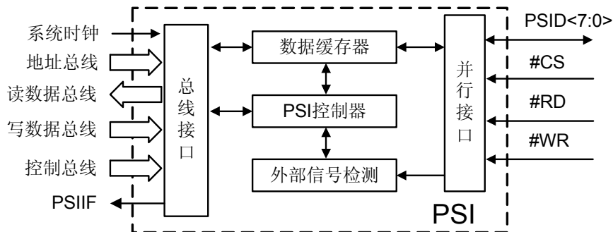
图 5-33 PSI 驱动模块框图
