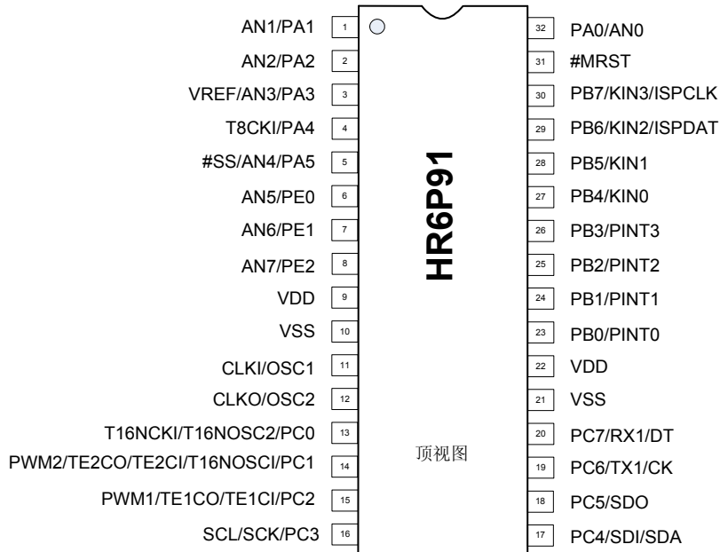
图 1-3 HR6P91/91H (SDIP32/SOP32) 顶视图
