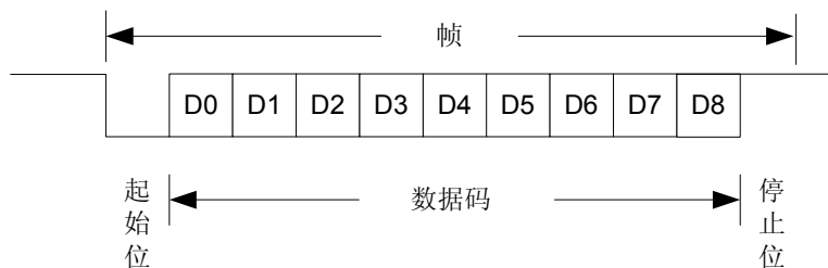
图 5-30 UART2 9 位数据格式
