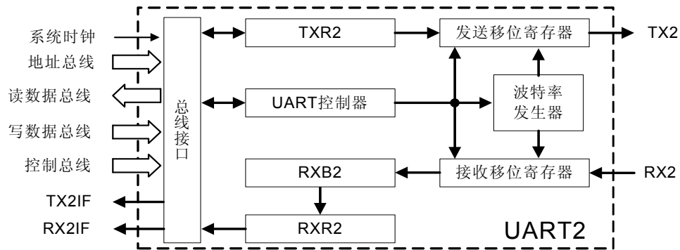
图 5-28 UART2 结构框图
