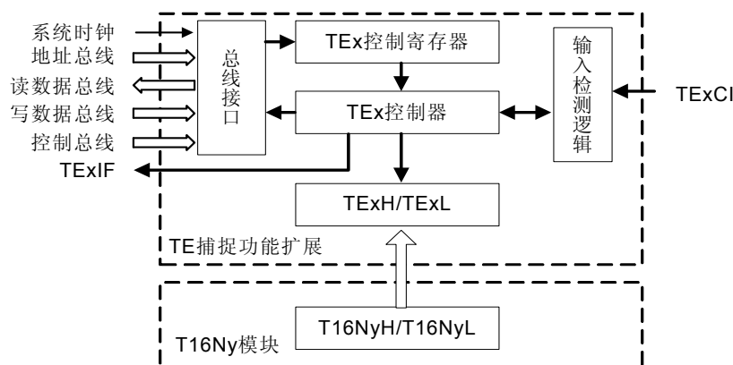
图 5-4 TE 捕捉功能扩展的内部结构图
