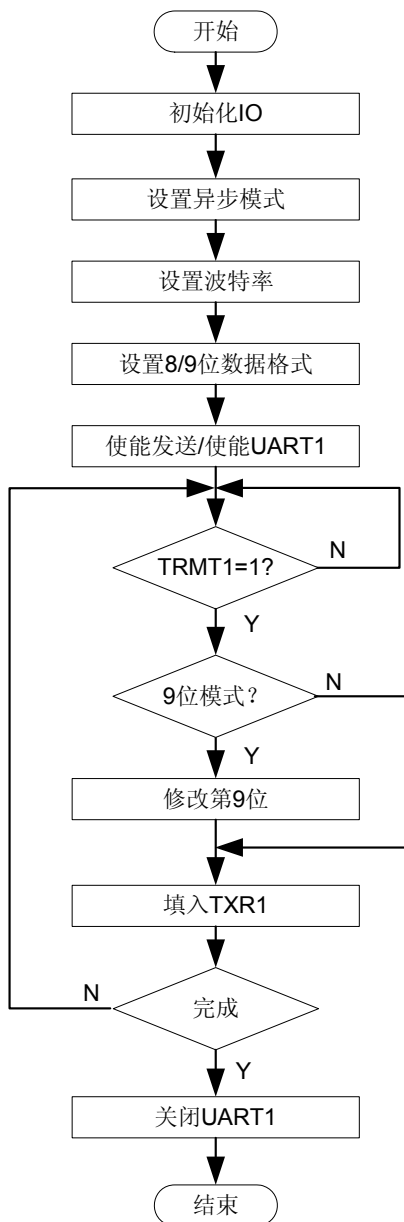
图 5-24 UART1 发送器流程图
