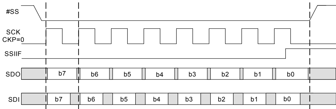
图 5-16 SPI 从动模式时序图 (CKP = 0)
