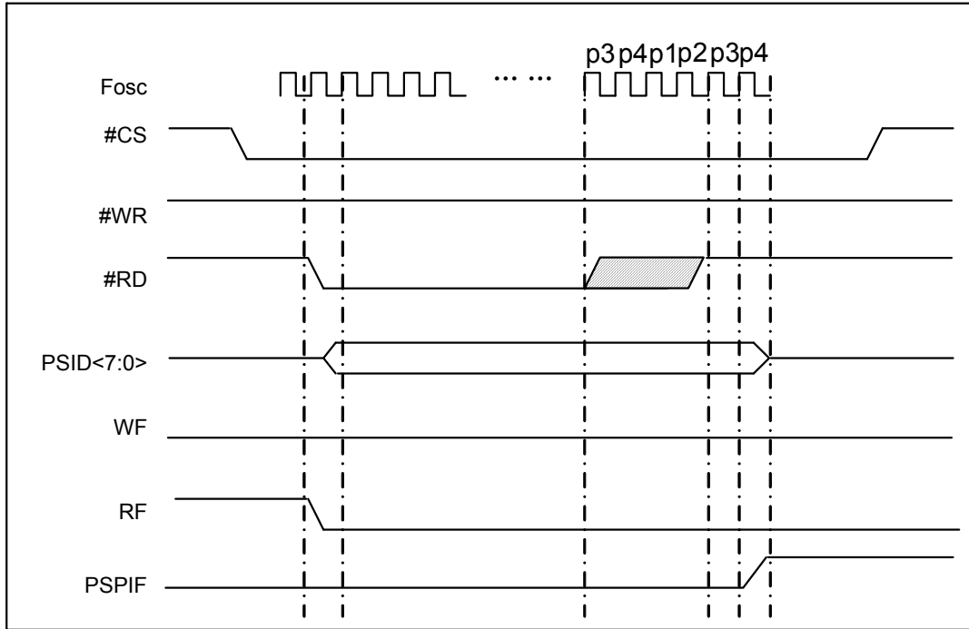
图 5-34 PSI 读出操作时序图
