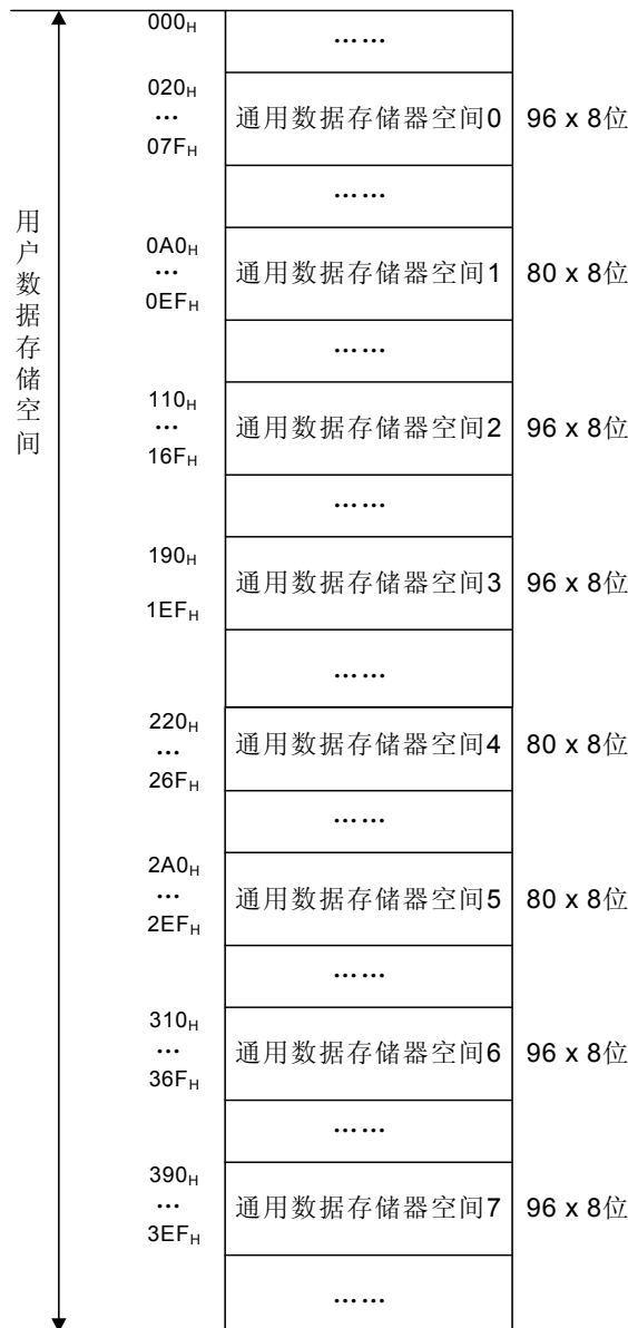
图 3-3 通用数据存储器地址映射示意图
