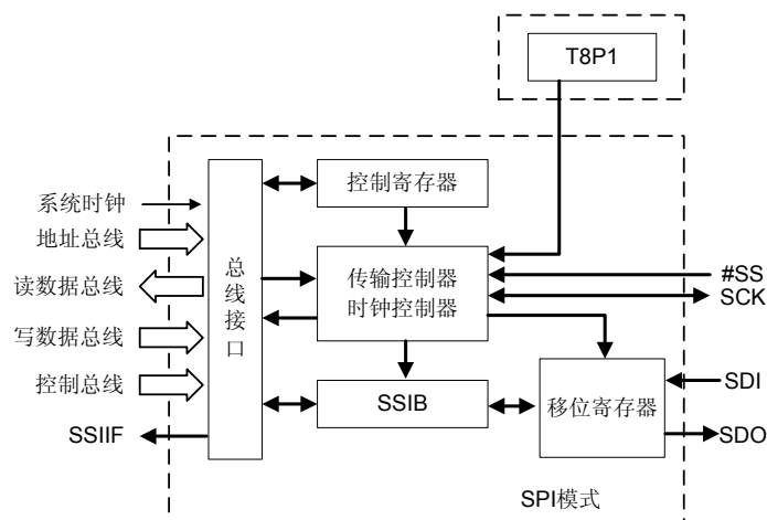
图 5-10 SPI 结构框图
