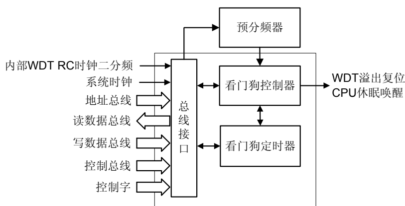
图 6-5 看门狗定时器示意图
