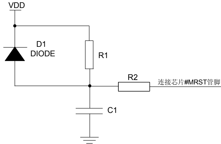
图 6-3 RC 复位电路
