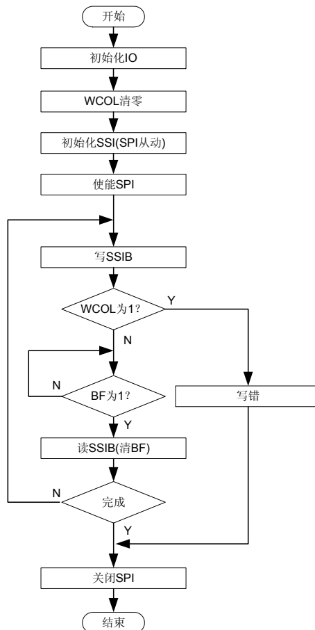
图 5-14 SPI 从动模式流程图
