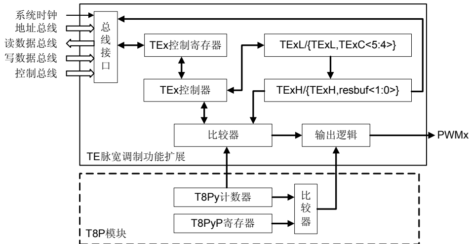
图 5-6 TE 在 PWM 功能扩展的内部结构图
