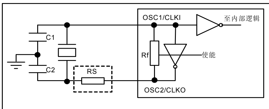
图 6-1 晶体/陶瓷振荡器模式（HS 模式）
