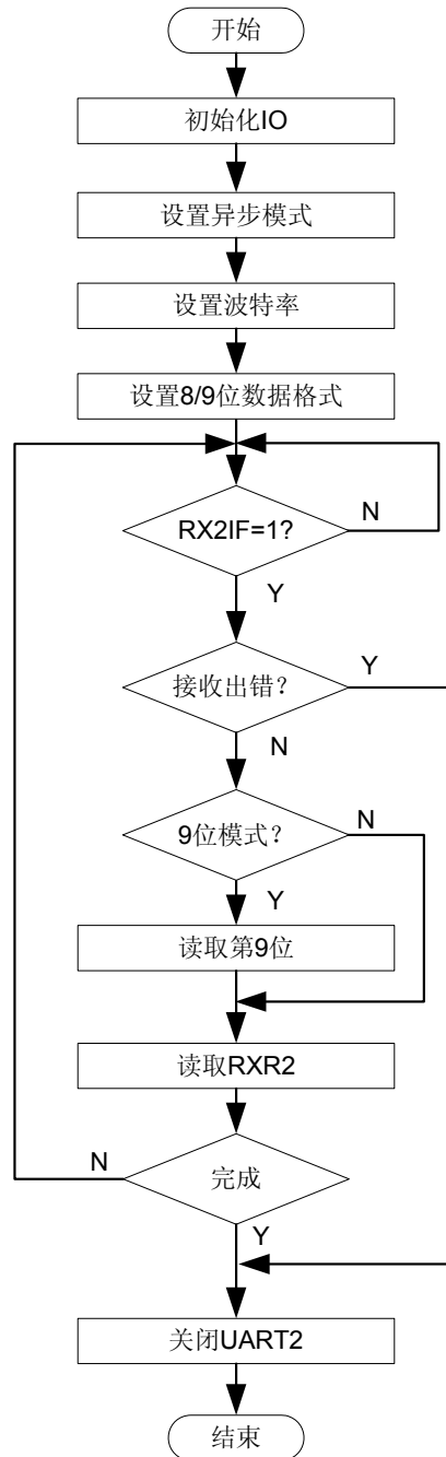
图 5-32 UART2 接收器流程图
