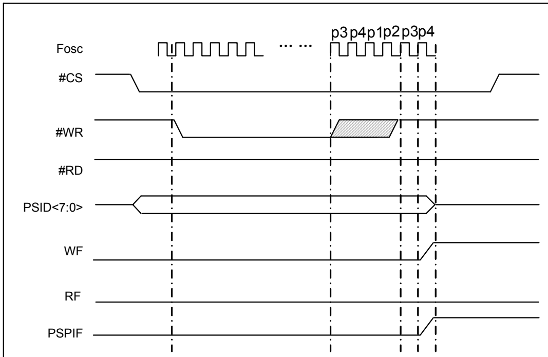
图 5-35 PSI 写入操作时序图
