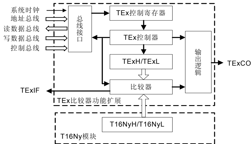
图 5-5 TE 比较器功能扩展的内部结构图
