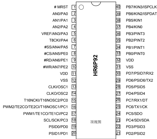
图 1-4 HR6P92/92H (DIP40) 顶视图
