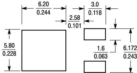
DPAK
