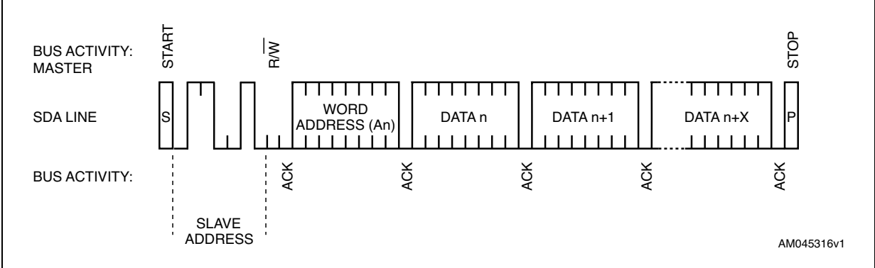
图 9. WRITE( 写 ) 模式序列
