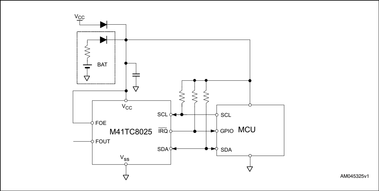
图 4. 硬件接线图
