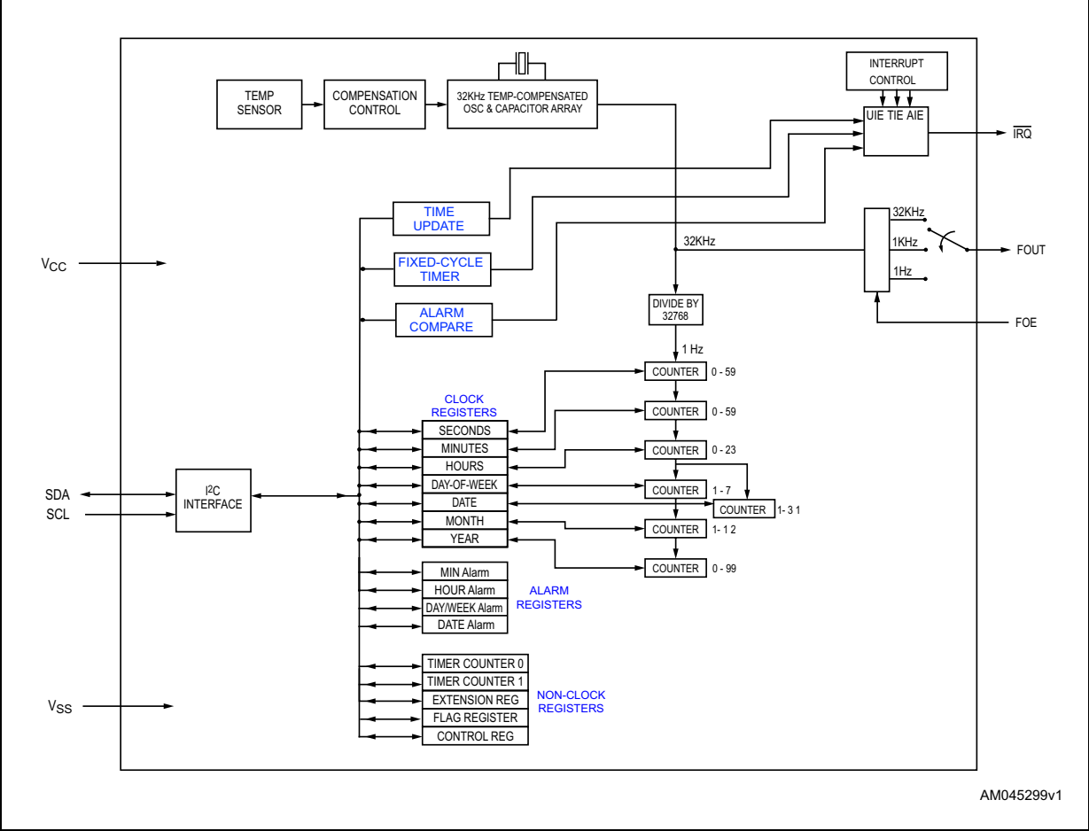
图 3. 框图
