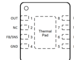
DFNW8 3x3, 0.65P CASE 507AD
